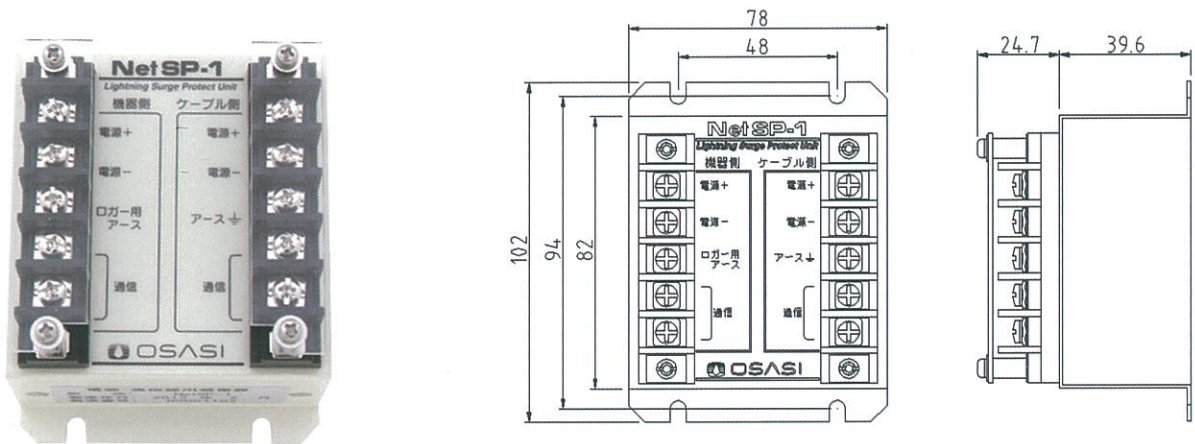
【機器構成例】
